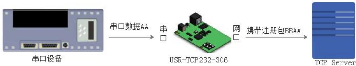
图 64. 数据携带注册包
