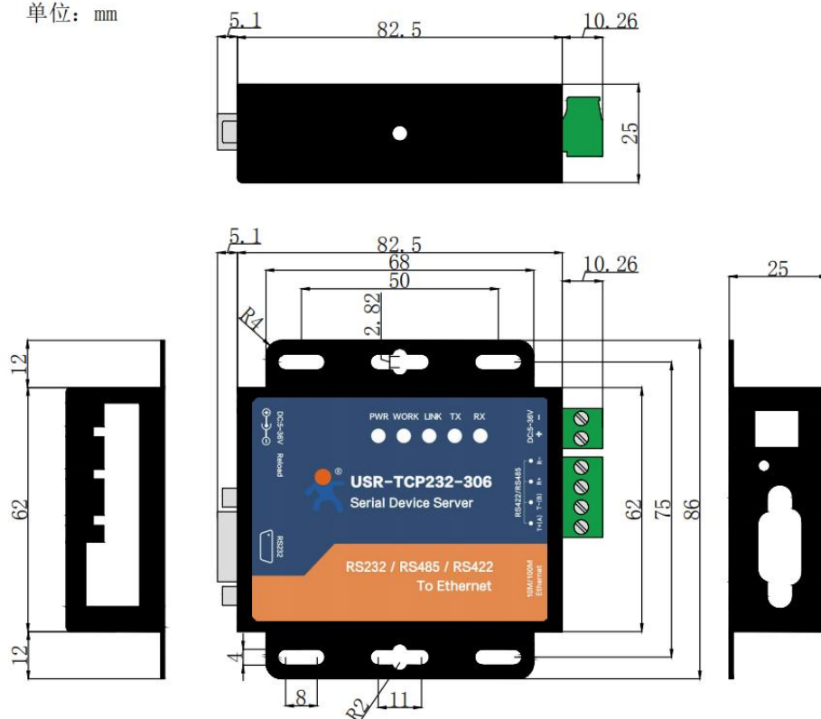
图 3. USR-TCP232-306 尺寸图
