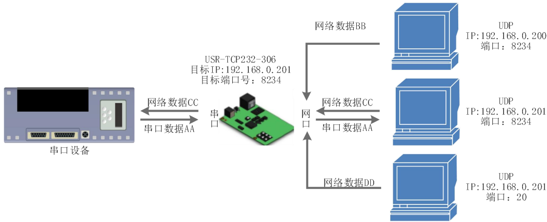
图 21. UDP Client 模式说明
