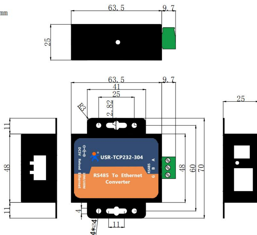
图 2. USR-TCP232-304 尺寸图
