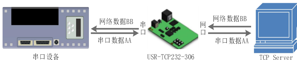
图 13. TCP Client 模式说明
